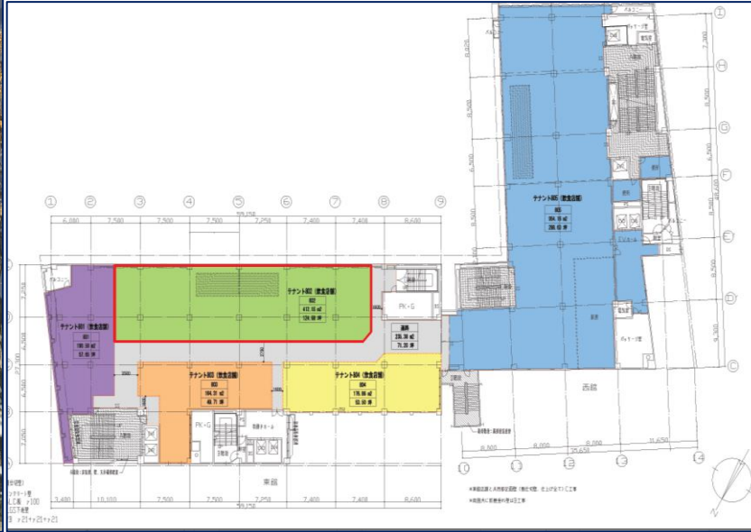
地上8階802区画
